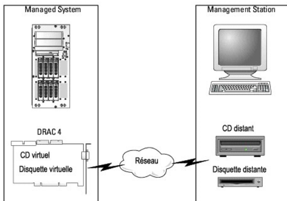
Figure 8-1. Architecture globale d'un média virtuel
